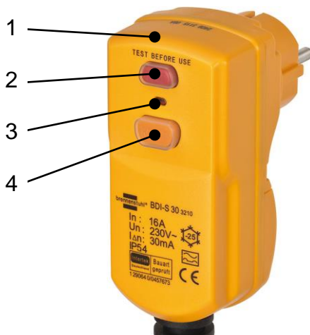
Рис. 4.2. Общий вид штепсельного разъёма, совмещённого с УЗО
